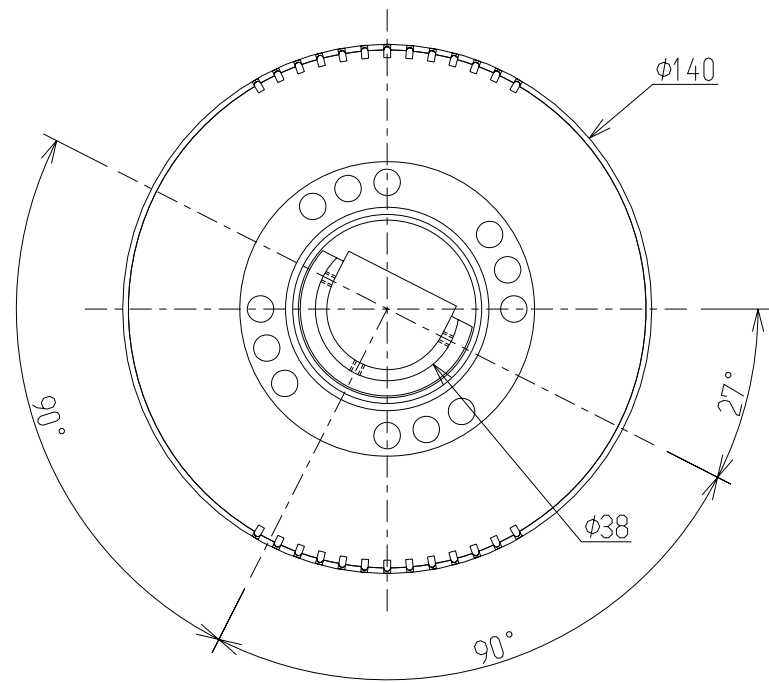
A 矢視図
