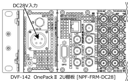
棚板 (DC28V電源用棚板) 背面
