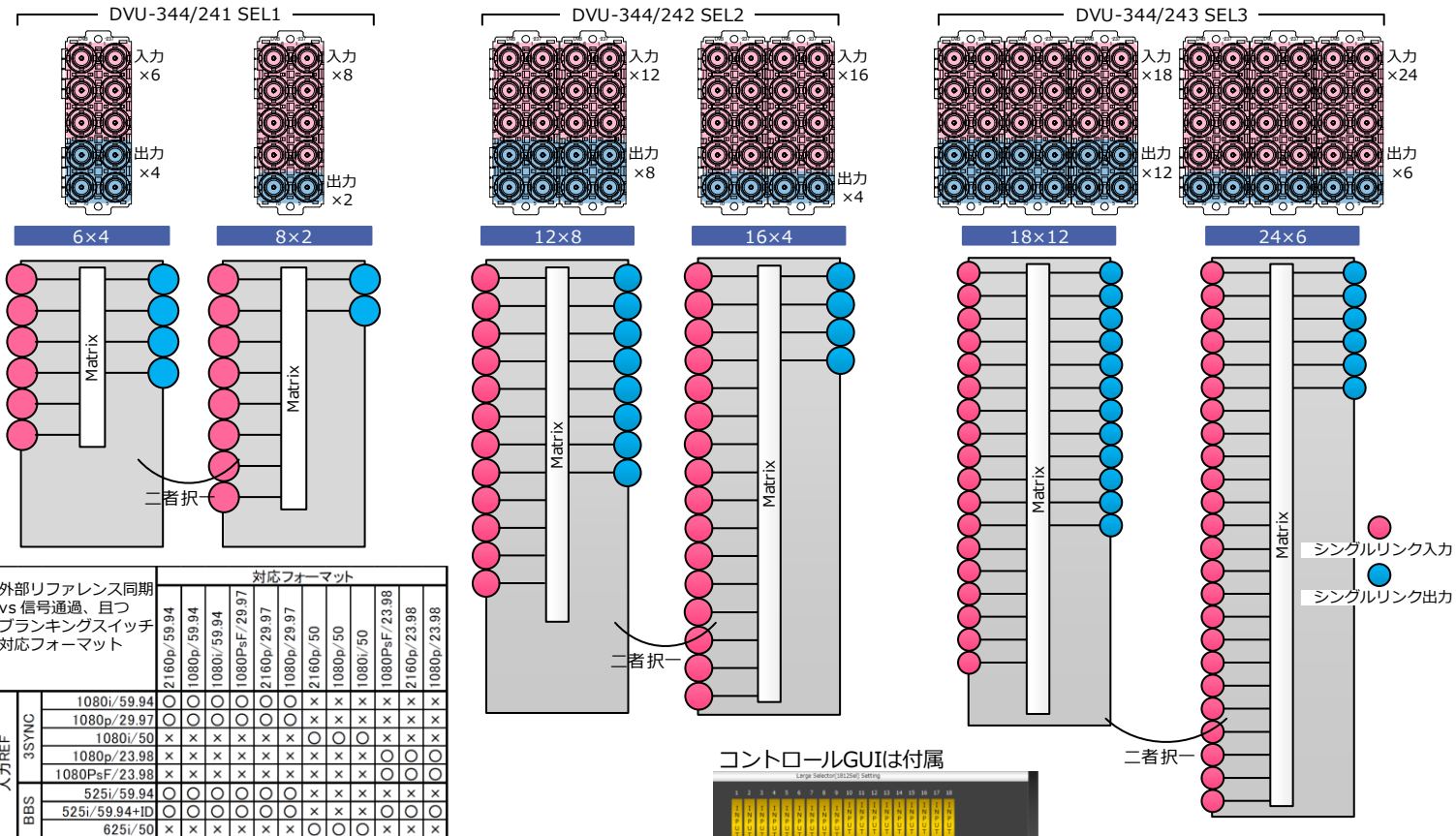
Rear module : 1スロット10コネクタ : DVB-241 NPF-SEL1-REAR 2スロット20コネクタ : DVB-242 NPF-SEL2-REAR 3スロット30コネクタ : DVB-243 NPF-SEL3-REAR
