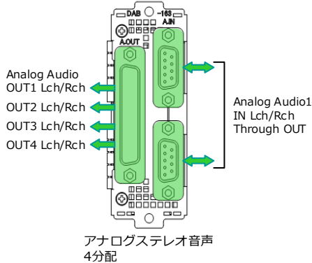
DAB-163 NPF-A-ADA4-REAR 背面コネクタI/F
