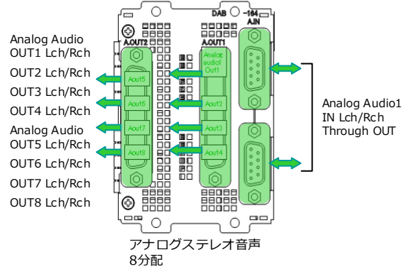
DAB-164 NPF-A-ADA8-REAR 背面コネクタI/F
