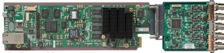
Front module : DVU-345 NPF-PROC
