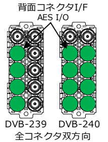
Rear module : DVB-239 NPF-AES4-REAR DVB-240 NPF-AES8-REAR
