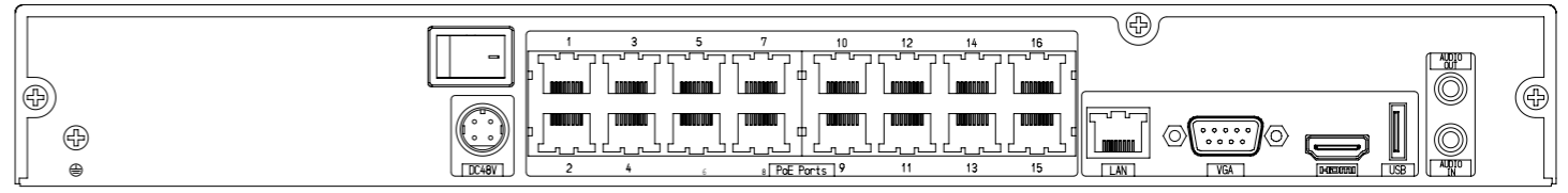
リアパネル詳細図 (S:1/2)
