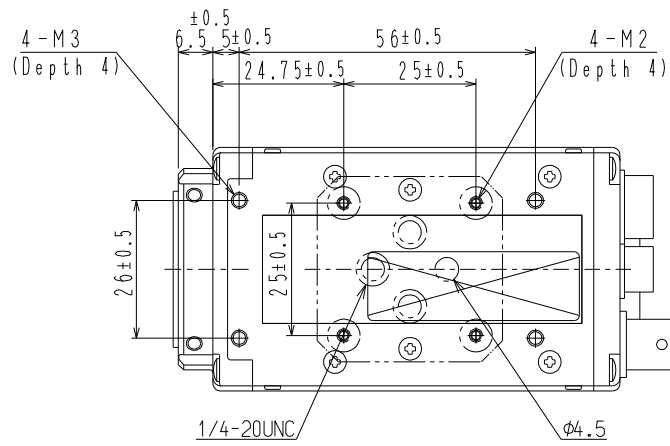
SKC-151 外觀圖
