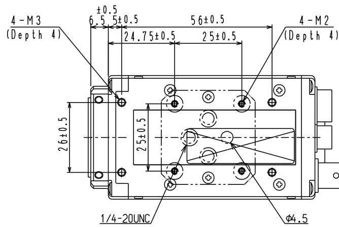
SKC-141CL 外觀圖
